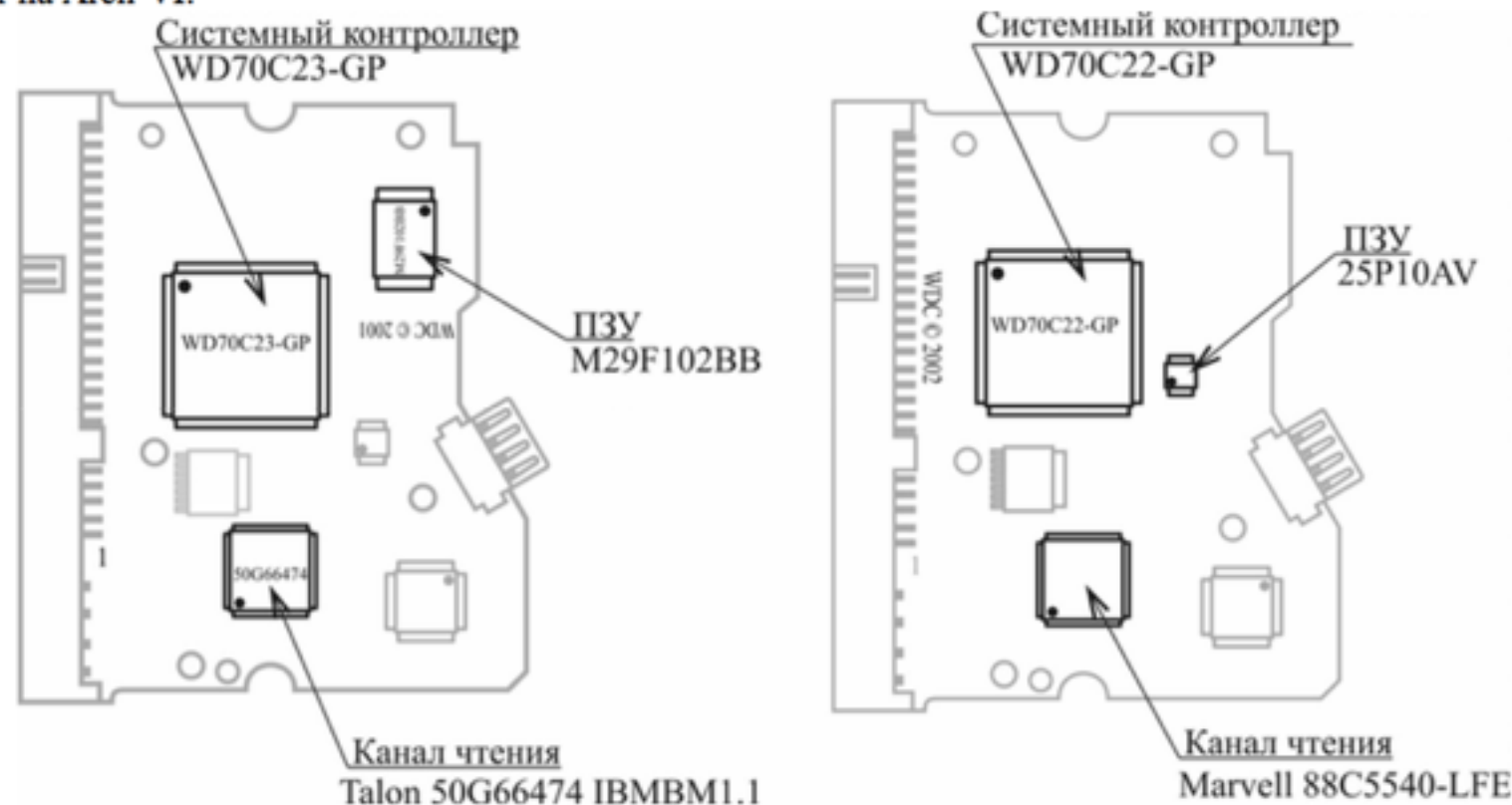
Схематический рисунок 2-х плат на WD70Cх
